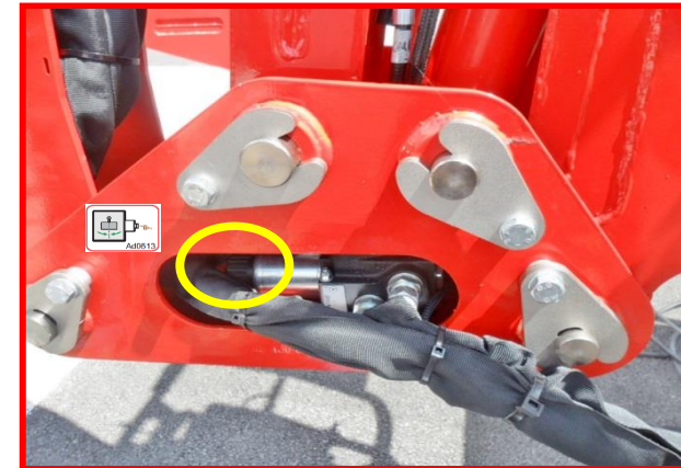
Figure 24 : curseur pour centrage de nacelle.
