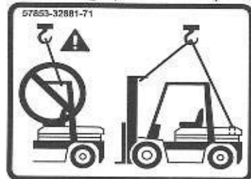
(1) Points de levage (mât extérieur)
